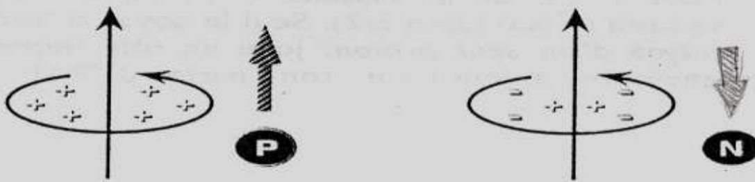
FIG. I-1. — Les neutrons comme les protons possèdent un moment magnétique lié à la distribution de charge de sous-particules positives et négatives en rotation : les quarks. Le moment magnétique du neutron est environ égal aux 2/3 de celui du proton.
